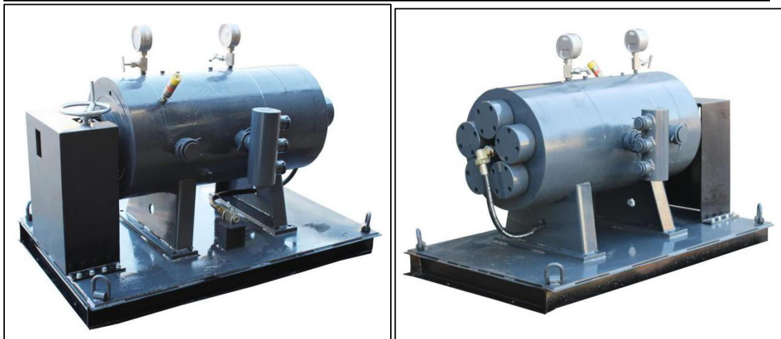
1-4、JSYL-GDX-HSD-KJ51/DN50(手动) 过滤装置结构图示：
