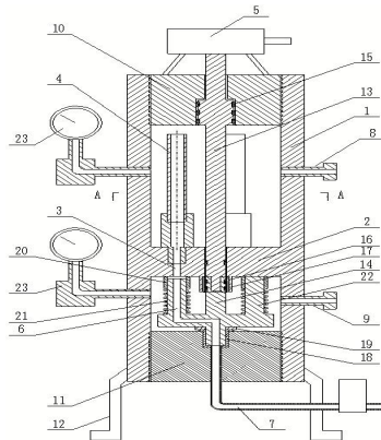
1-4、JSYL-GDX-HSD-KJ51/DN50(手动) 过滤装置结构图示：
