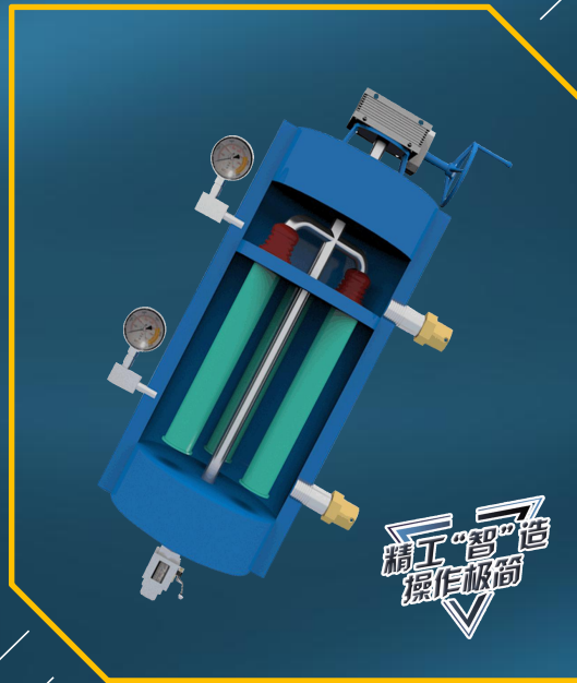
喷雾专用过滤器 剖面图
